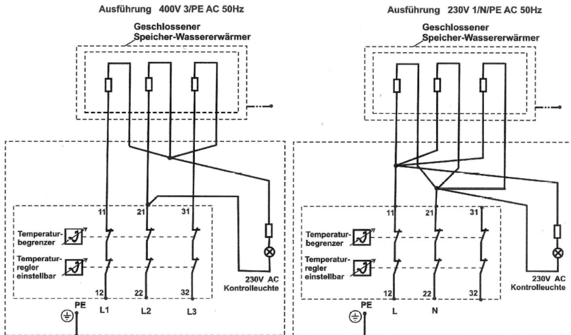
Schaltbild Einschraubheizkörper
